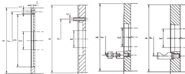
typ cylindryczny (DIN 6350) typ A i B (DIN 55026) typ C (DIN 55027) typ D (DIN 55029) type cylindrical (DIN 55026) type A and B (DIN 55026) type C (DIN 55027) type D (DIN 55029) mun (DIN 55026) mun A и B (DIN 55026) mun C (DIN 55027) mun D (DIN 55029)
