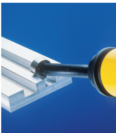
GRATOWNIK GT-KEYWAY Gratownik teleskopowy do fazowania krawędzi wewnętrznych GT-KEYWAY-BURR i zewnętrznych krawędzi kanałków o szerokości od 2,4 mm do 11 mm. EL1400GT
