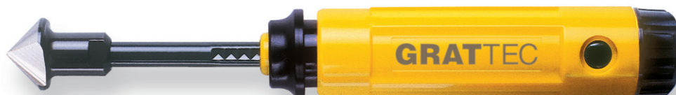
POGŁĘBIACZ GT Teleskopowy pogłębiacz stożkowy do pogłębiania i fazowania otworów. GT-COUNTERSINK Przydatny do głębiej położonych otworów. EL1300GT
