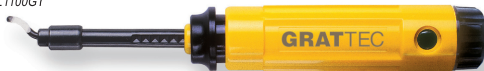
GRATOWNIK GT "B" Uniwersalny gratownik teleskopowy z ostrzami typu "B" GT "B" SET o średnicy trzpienia 2,6 mm. EL1100GT
